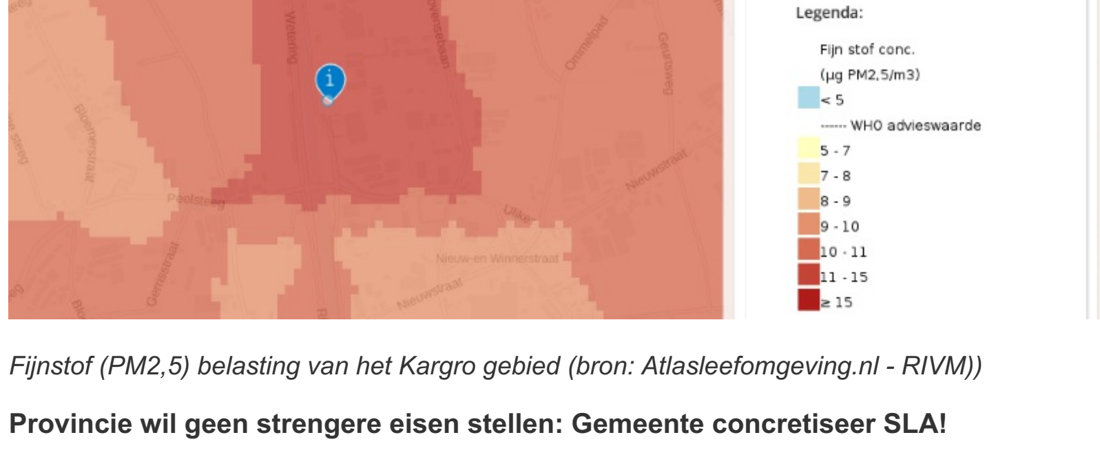
Fijnstof (PM2,5) belasting van het Kargro gebied (bron: Atlasleefomgeving.nl - RIVM)
